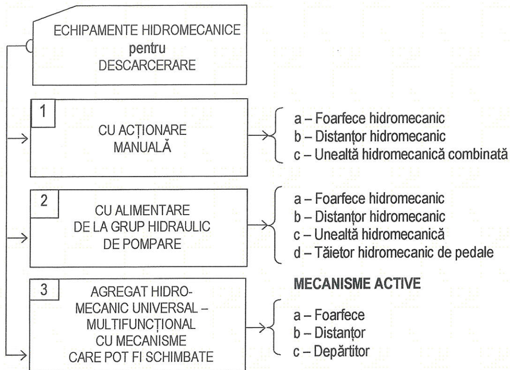
Schema structurală 1
