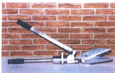
Fig. 1 b. Distanțor hidraulic
